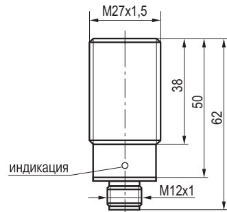
Габаритный чертеж
